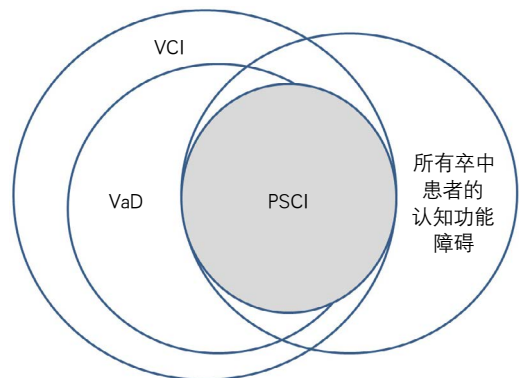
图1 VCI和PSCI以及常见定义的关系图
